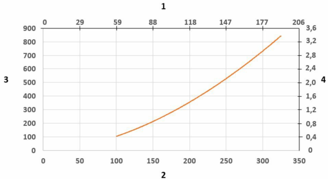
Drukverlies diagram: 1) X- As: Luchthoeveelheid (cfm) 2) X- As: Luchthoeveelheid (m³/h) 3) Y-Axis: Drukverlies (Pa) 4) Y-Axis: Drukverlies (in. wg.)
