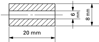
(2) Collare fissaggio (8 × 6)
