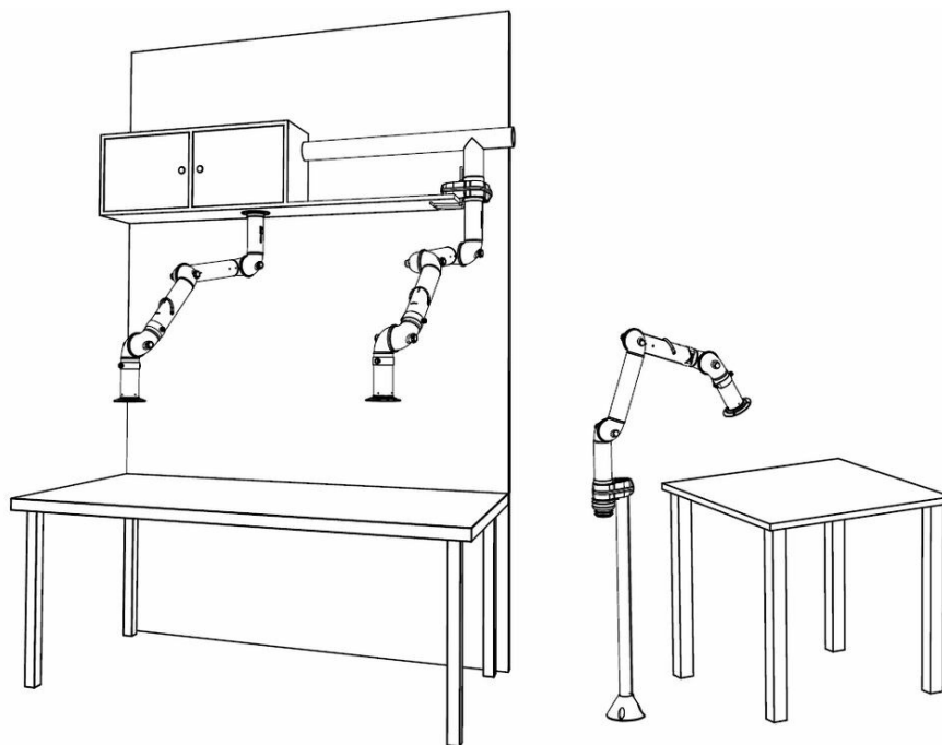
Andere montage voorbeelden: Links: Over tafel cabinet montage met FX2-Omhoog/Beneden-Door arm met de volgende accessoires: -FX2-Tafelbeugel kit Rechts: Vloer montage met FX2-Omhoog-Laag arm en de volgende accessoires: -FX-Standaard beugel -FX-Cut2fit verlenging-L1100
