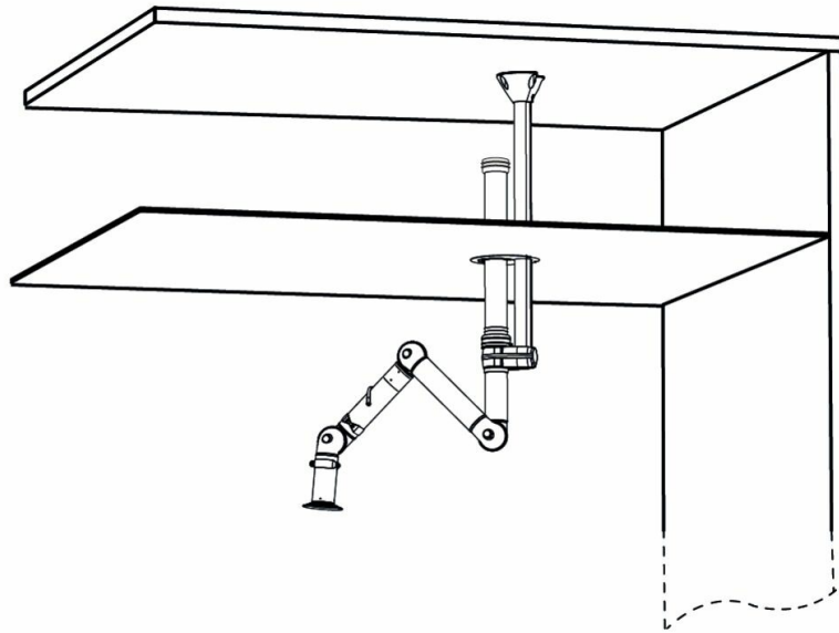
Plafond montage voorbeeld: Links: FX2-Omhoog-Laat arm met de volgende accessoires: -FX-Standaard beugel -FX-Cut2fit verlenging-L1100 -FX2-Alu leiding -FX2-Leiding connector-ESD/EX-D100 -FX-Plafond afdekplaat
