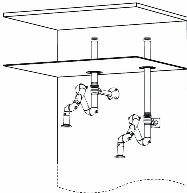
Muur bevestiging voorbeelden: Links: FX2-Omhoog-PLUS arm met volgende accessoires: -FX2-Beugel kit-D-50/75/100-L500 - FX2-plafond afdekplaat-PLUS -Alu leiding -Leiding connector-ESD/EX-D100 Rechts: Omhoog-Laat arm met de volgende accessoires: -FX2-Muur beugel kit-plat-L190-Zwart -FX2-Plafond afdekplaat-PLUS -FX2-Alu leiding -FX2-Leiding connector-ESD/EX-D100
