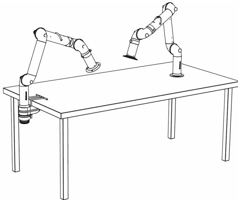
Tafel montage voorbeelden: Links: FX2-Beneden-Laag arm met de volgende accessoires: -FX2-Tafel beugel kit-D-50/75/100 Rechts: FX2-Beneden-door- arm
