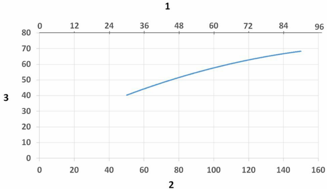
Gelduïdsniveau diagram: 1) X- As: Luchthoeveelheid (cfm) 2) X- As: Luchthoeveelheid (m³/h) 3) Y-As: Gelduïdsniveau (dBA)
